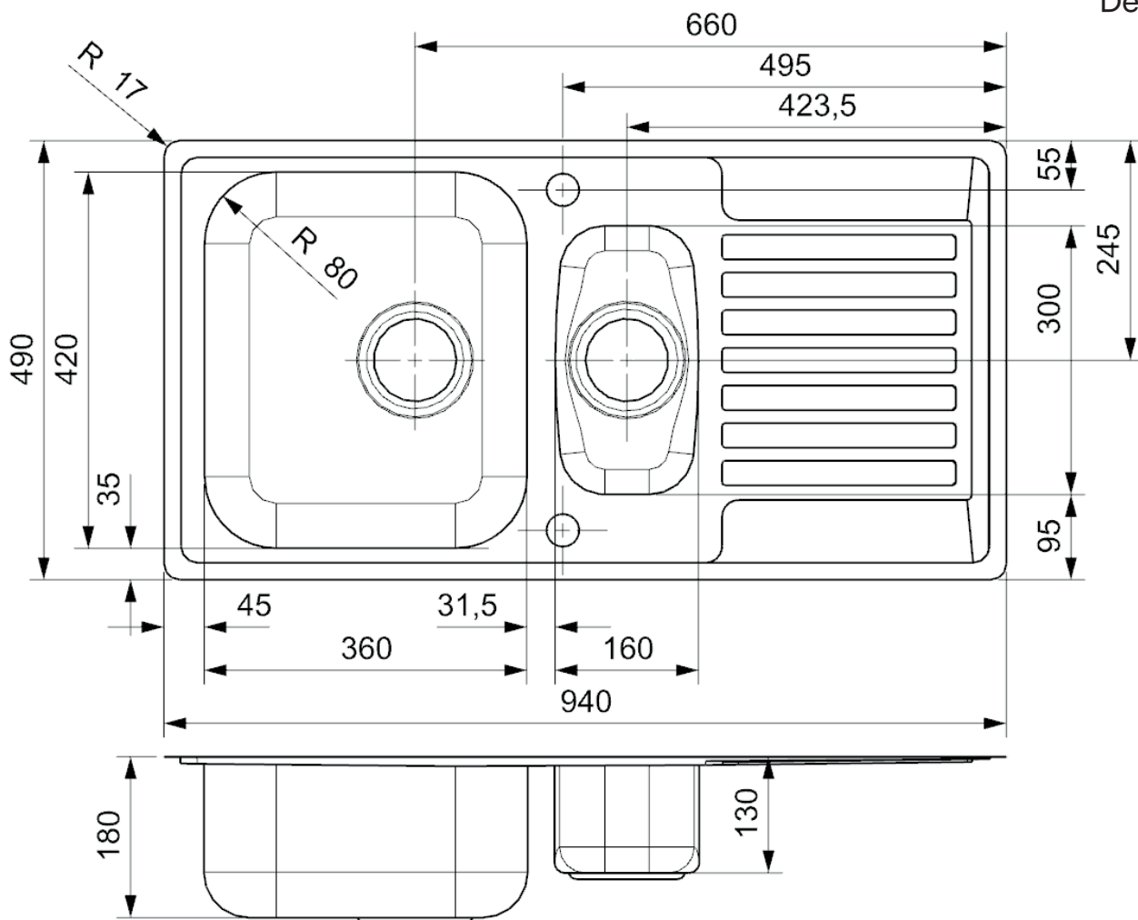
Detalje A
